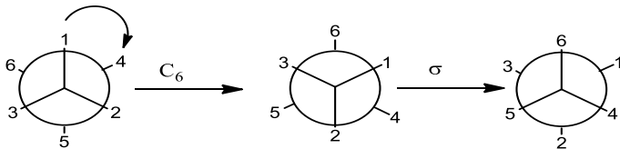
۱۷- شکل: نیومن جوړښت دی کوم چې د ایتان مرکب دی. دمحوری دوران انعکاس عمل ښيي
