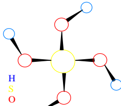
۱۶- شکل: [H_2SO_4]^{-2} مالیکول دی
