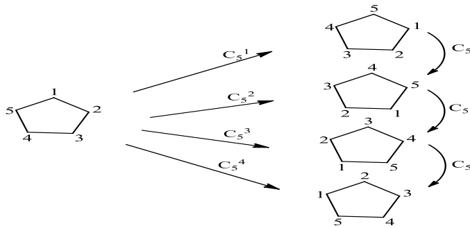
۱۰- شکل: ساپکلو پنتاډاين آيون د ساده محوری دوران عمل ښيي
