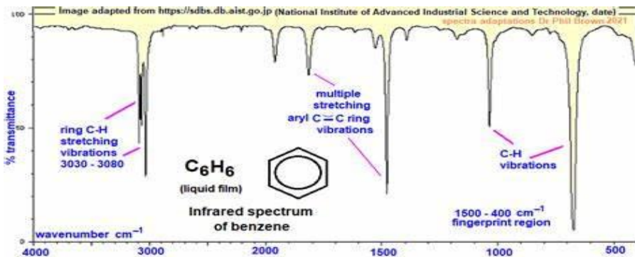
۴- شکل: د بنزين طيف
