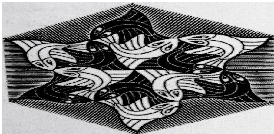
۲- شکل: د دائر ماهی شکل
