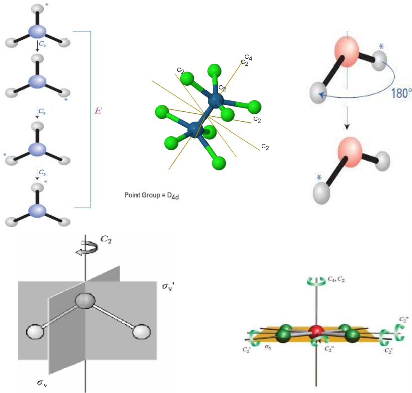
۶- شکل: هغه مالیکولونه چې د تقارن څخه برخورداره دي
