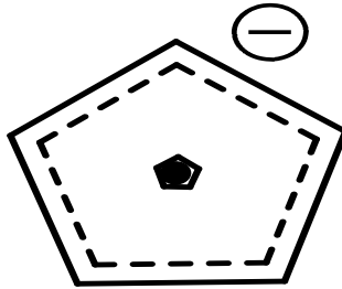
۹- شکل: د سا يکلو پنتاډاين آيون دی
