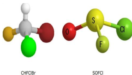
۲۱- شکل: یاد مالیکولونه واحد عمل ښيي
