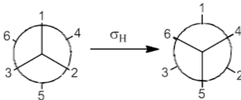
۱۸- شکل: د نیومن جوړښت کې دانعکاس عمل د افقی صفحه په واسطه
