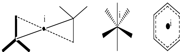
۲۰- شکل: نوموړې شکلونه د تقارن مرکز ښيي
