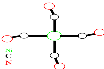
۱۵- شکل: د [Ni(CN)_4]^{2-} مالیکول دی
