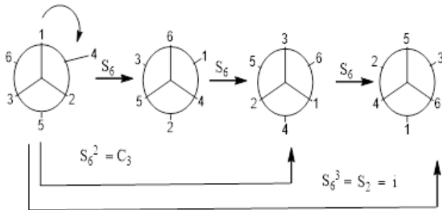
۱۹- شکل: دمحوري دوران انعکاس ښيي
