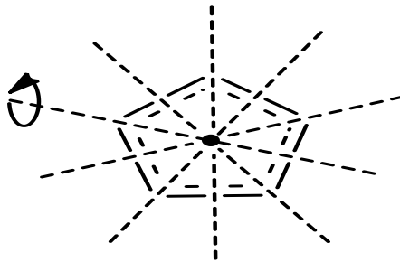
۱۱- شکل: نوموړی شکل د C_2 محور ښيي
