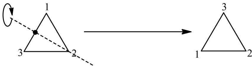
۷- شکل: د BH_3 مالیکول دی د تقارن عملیه ښيي
